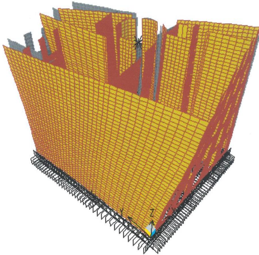
Şekil 6. 3. Mod Şekli T_3=0.09s
