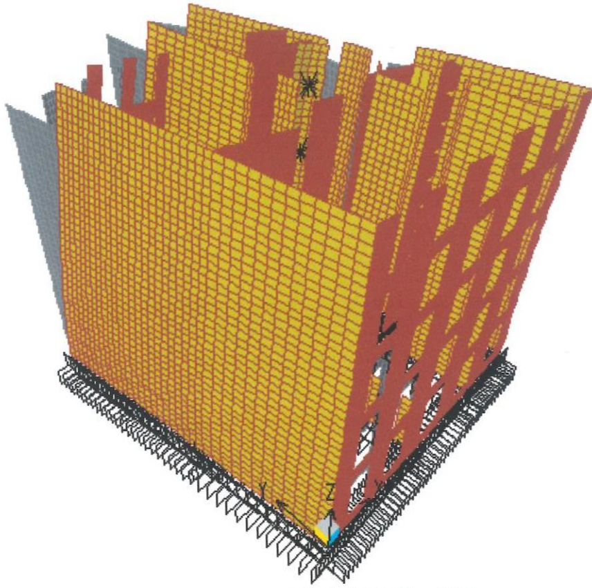
Şekil 4. 1. Mod Şekli T_1=0.28s
