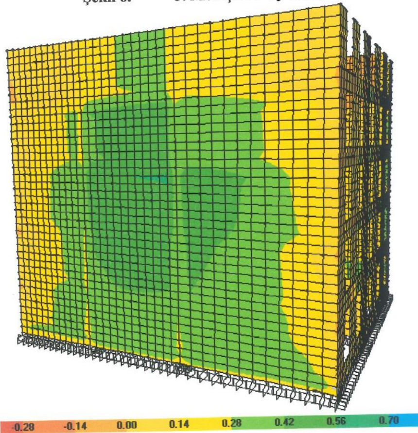
Şekil 7. Y Yönünde Deprem Durumu 1 Aksı Duvarı Kayma Gerilmesi Dağılımı
