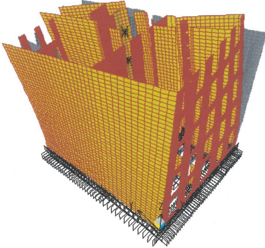
Şekil 4. 1. Mod Şekli T_1=0.28s
